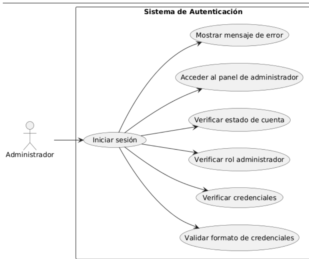
Diagrama De Caso de Uso CU – 02
